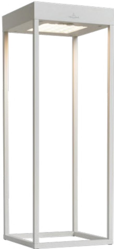
CANNES | 96910 18,5 x 18,5 cm, h 50 cm 2,2 W LED, 150lm, IP 65, 2700K & 3000K outdoorischleuchte aluminium weiß, inkl. dimmer, 2 farbttemperaturen, dämmerungssensor, hybrid ladetechnik: solar & USB outdoor table lamp aluminum white, incl. dimmer, 2 colour temperatures, twilight sensor, hybrid charging: solar & USB lampe de table d'extérieur aluminium blanc, avec variateur, 2 températures de couleur, capteur cré- pusculaire, charge hybride: solaire & USB
